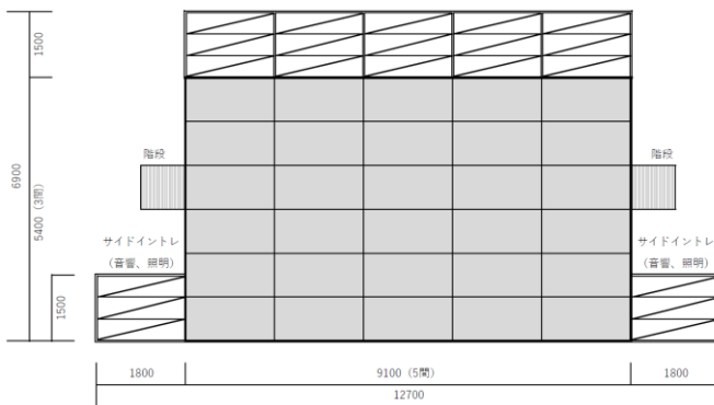
ステージ寸法 塗りつぶし部がステージ立ち部
